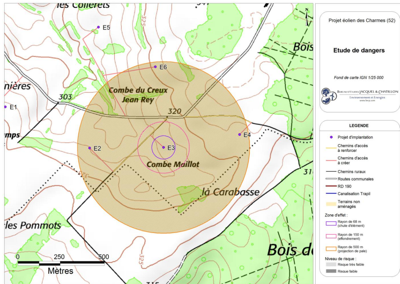
Carte 30 : Éolienne n°3 – Risques liés à l'effondrement de l'éolienne, à la chute d'élément de l'éolienne, et à la projection de pale ou de fragment de pale (Source : BE Jacquiel et Chatillon)
