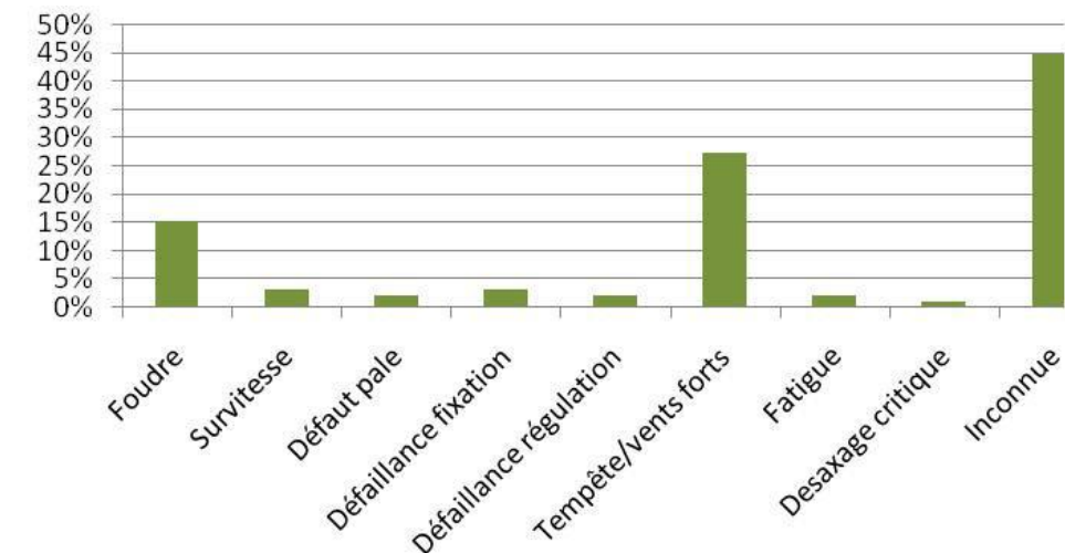
Figure 8 : Répartition des causes premières de rupture de pale (Source : INERIS)
