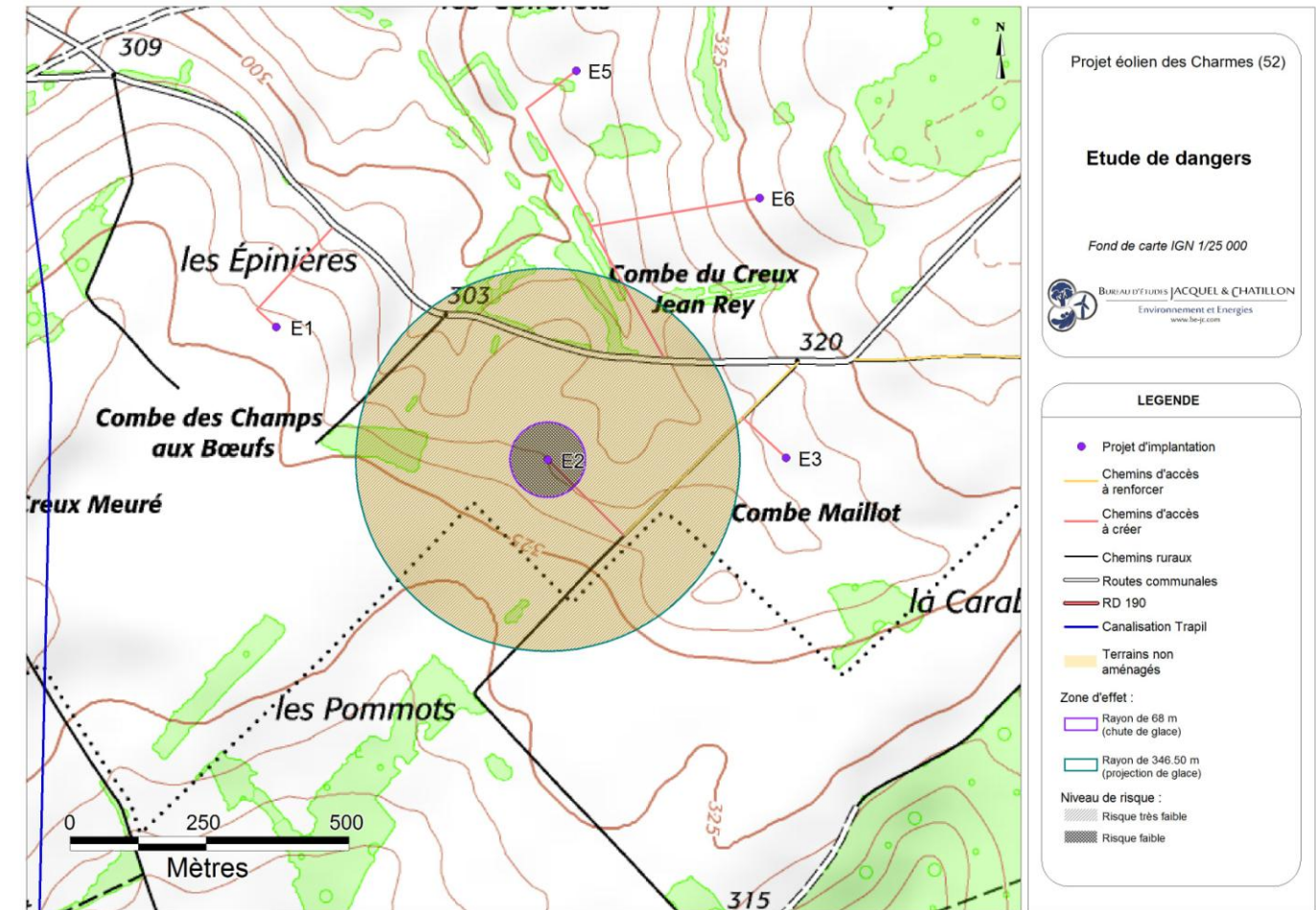
Carte 29 : Éolienne n°2 – Risques liés à la chute et à la projection de glace (Source : BE Jacquel et Chatillon)
