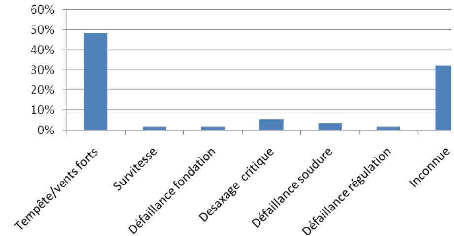
Figure 7 : Répartition des causes premières d'effondrement (Source : INERIS)
