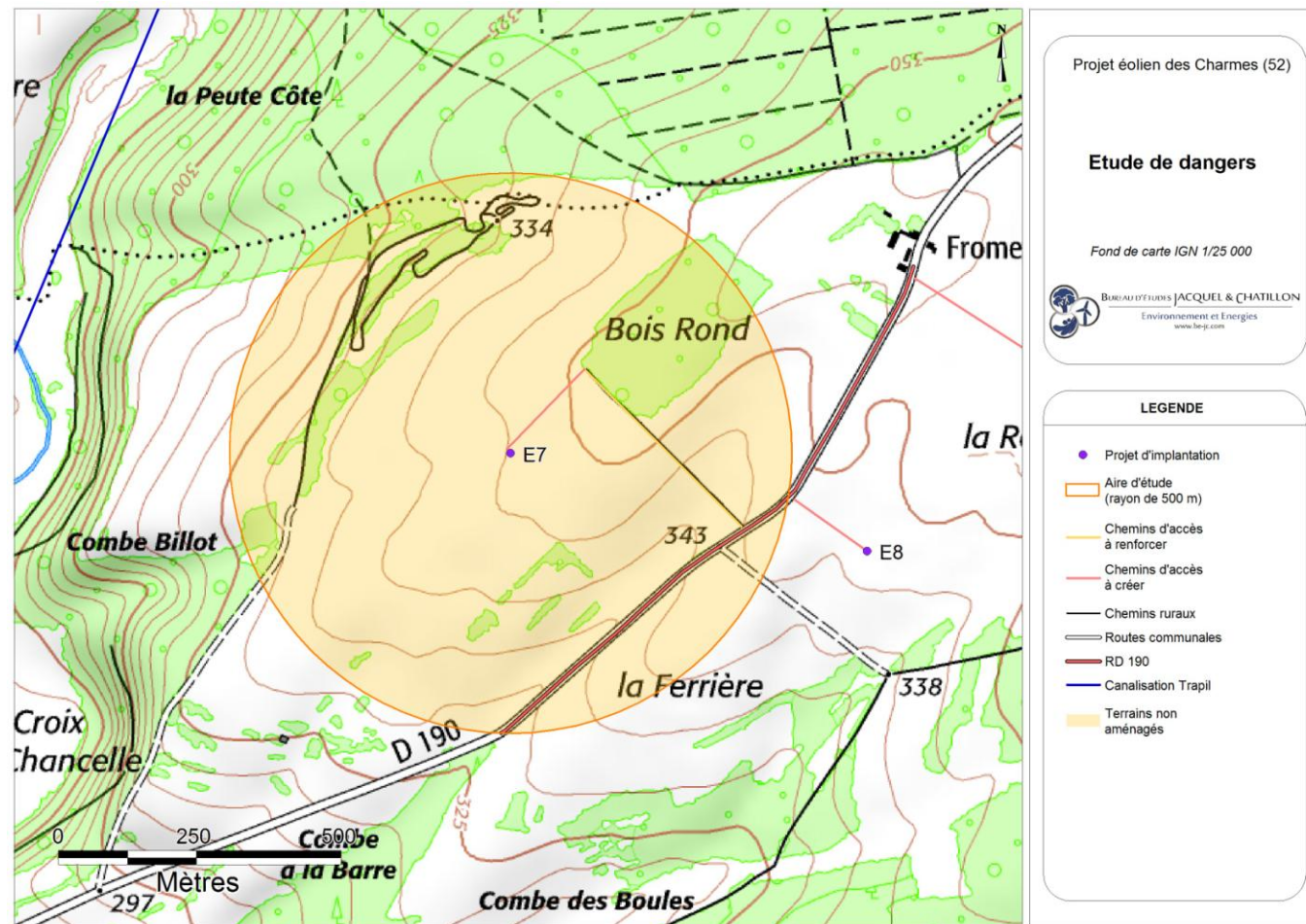
Carte 21 : Éolienne n°7 – Zones à enjeux (Source : BE Jacquel et Chatillon)
