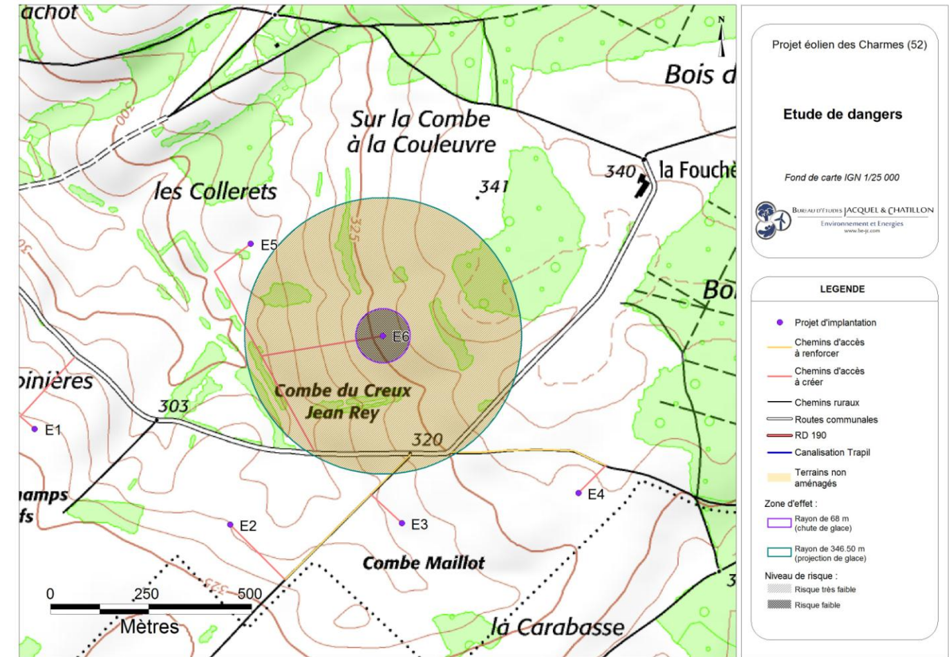
Carte 37 : Éolienne n°6 – Risques liés à la chute et à la projection de glace (Source : BE Jacquel et Chatillon)
