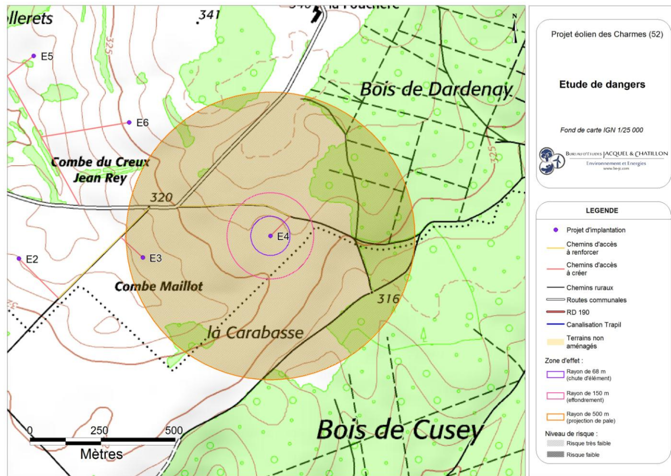
Carte 32 : Éolienne n°4 – Risques liés à l'effondrement de l'éolienne, à la chute d'élément de l'éolienne, et à la projection de pale ou de fragment de pale (Source : BE Jacquel et Chatillon)
