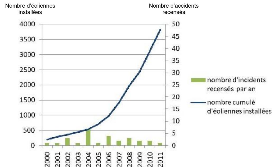
Figure 10 : Évolution du nombre d'incidents annuels en France et nombre d'éoliennes installées (Source : INERIS)
