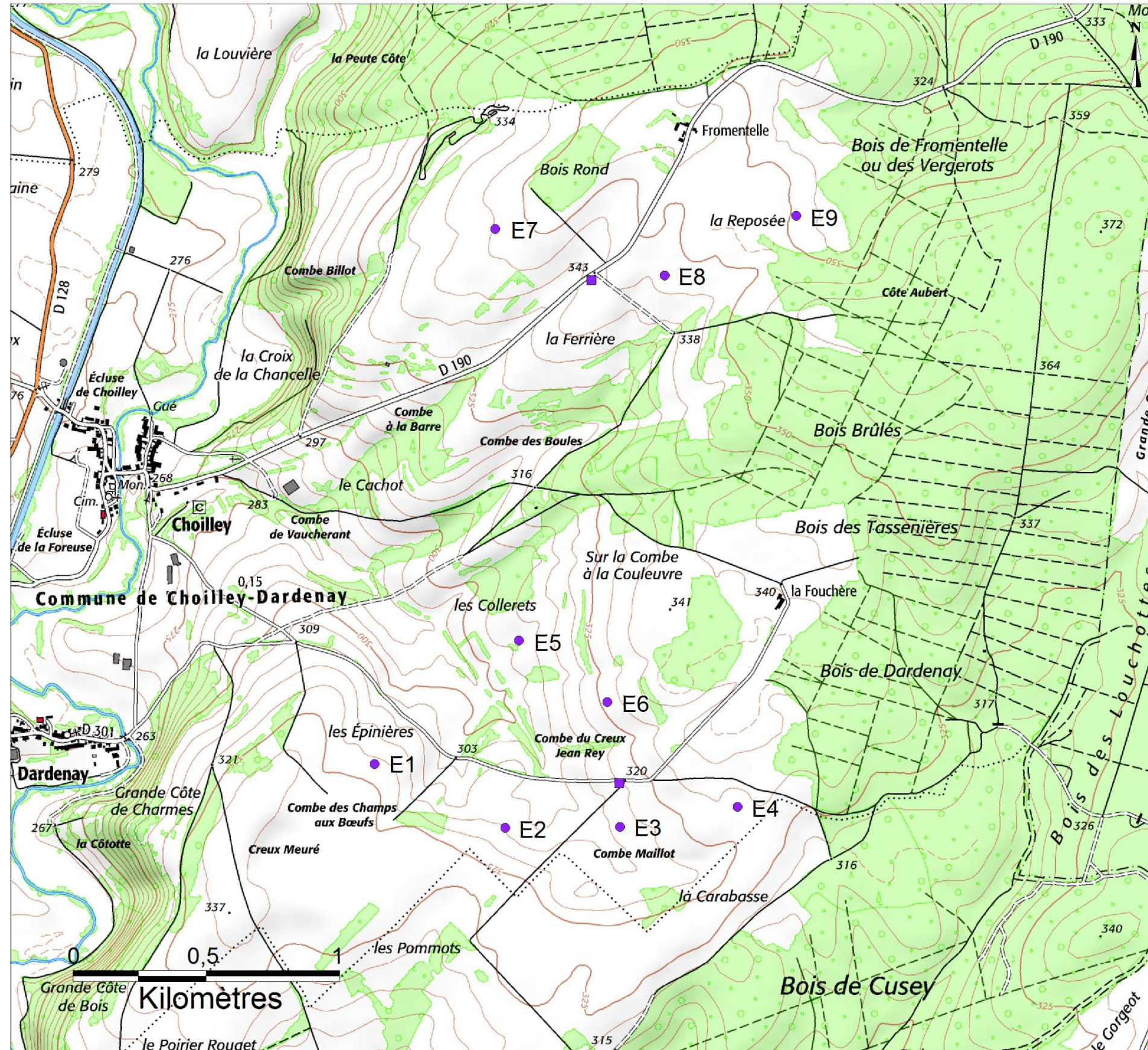
Carte 24 : Configuration de l'installation (Source : BE Jacquel et Chatillon)
