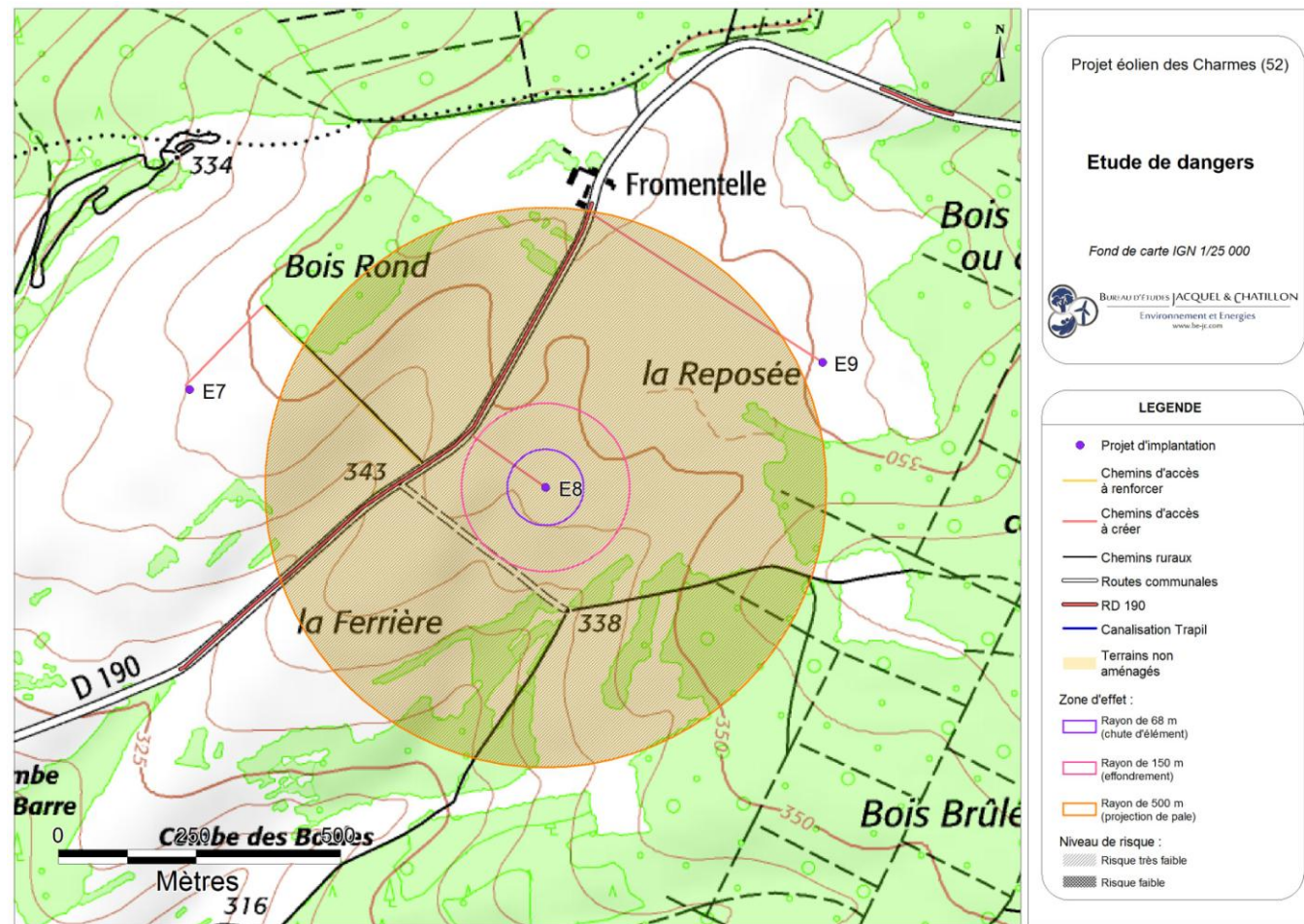
Carte 40 : Éolienne n°8 – Risques liés à l'effondrement de l'éolienne, à la chute d'élément de l'éolienne, et à la projection de pale ou de fragment de pale (Source : BE Jacquel et Chatillon)
