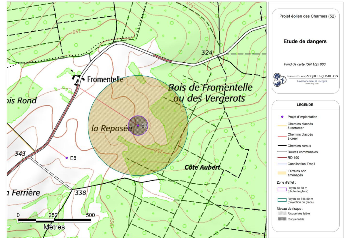
Carte 43 : Éolienne n°9 – Risques liés à la chute et à la projection de glace (Source : BE Jacquiel et Chatillon)
