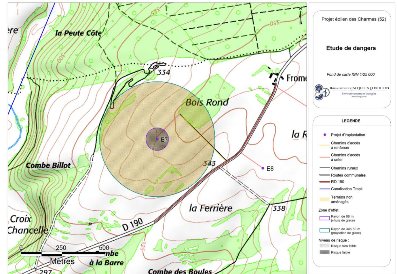
Carte 39 : Éolienne n°7 – Risques liés à la chute et à la projection de glace (Source : BE Jacquiel et Chatillon)
