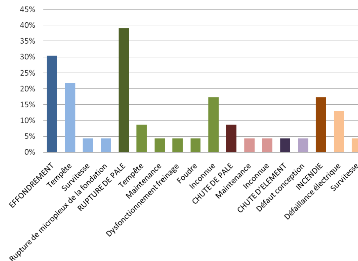
Figure 5 : Répartition des événements accidentels et de leurs causes premières sur le parc éolien français entre 2000 et 2011 (Source INERIS)
