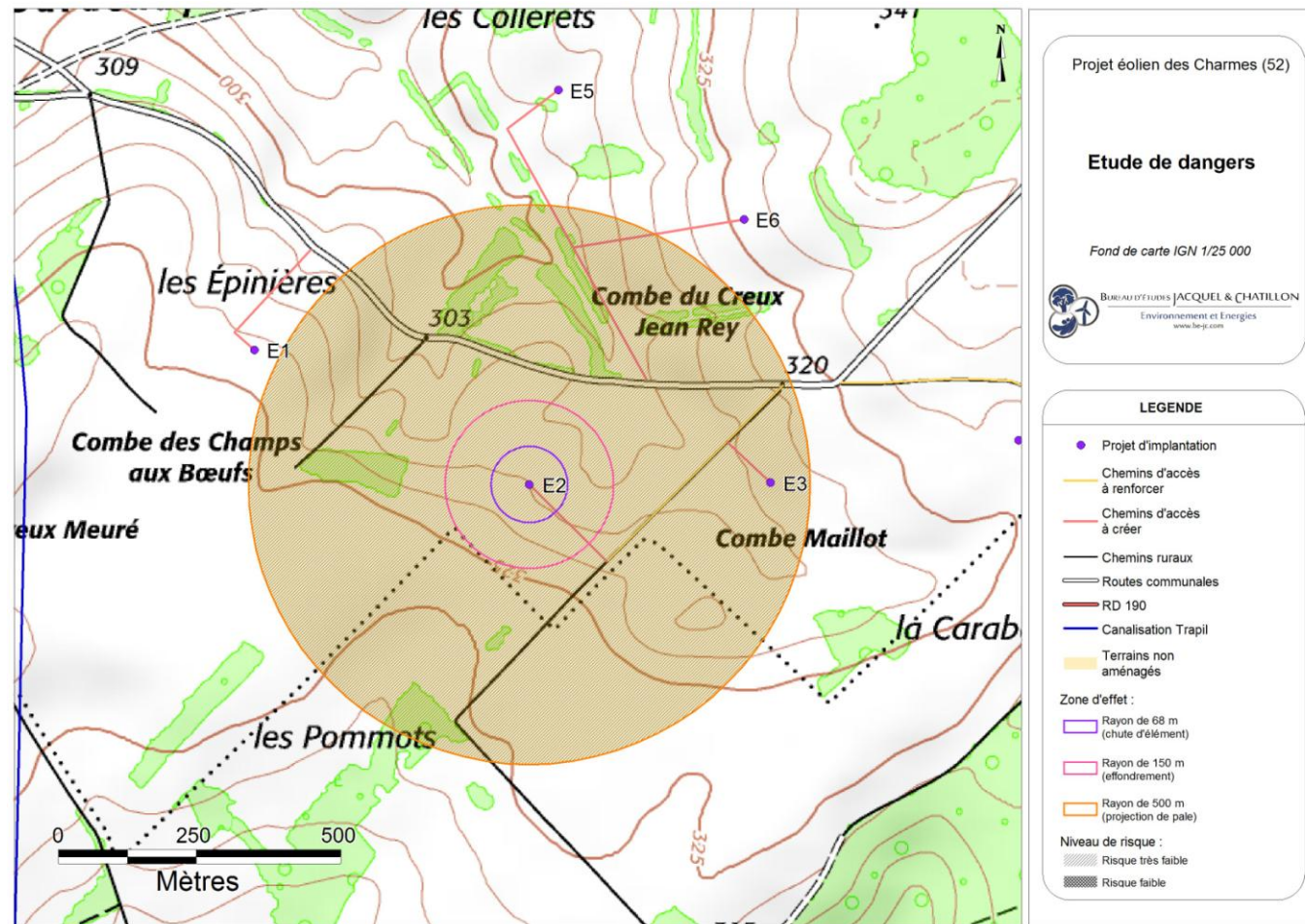
Carte 28 : Éolienne n°2 – Risques liés à l'effondrement de l'éolienne, à la chute d'élément de l'éolienne, et à la projection de pale ou de fragment de pale (Source : BE Jacquel et Chatillon)
