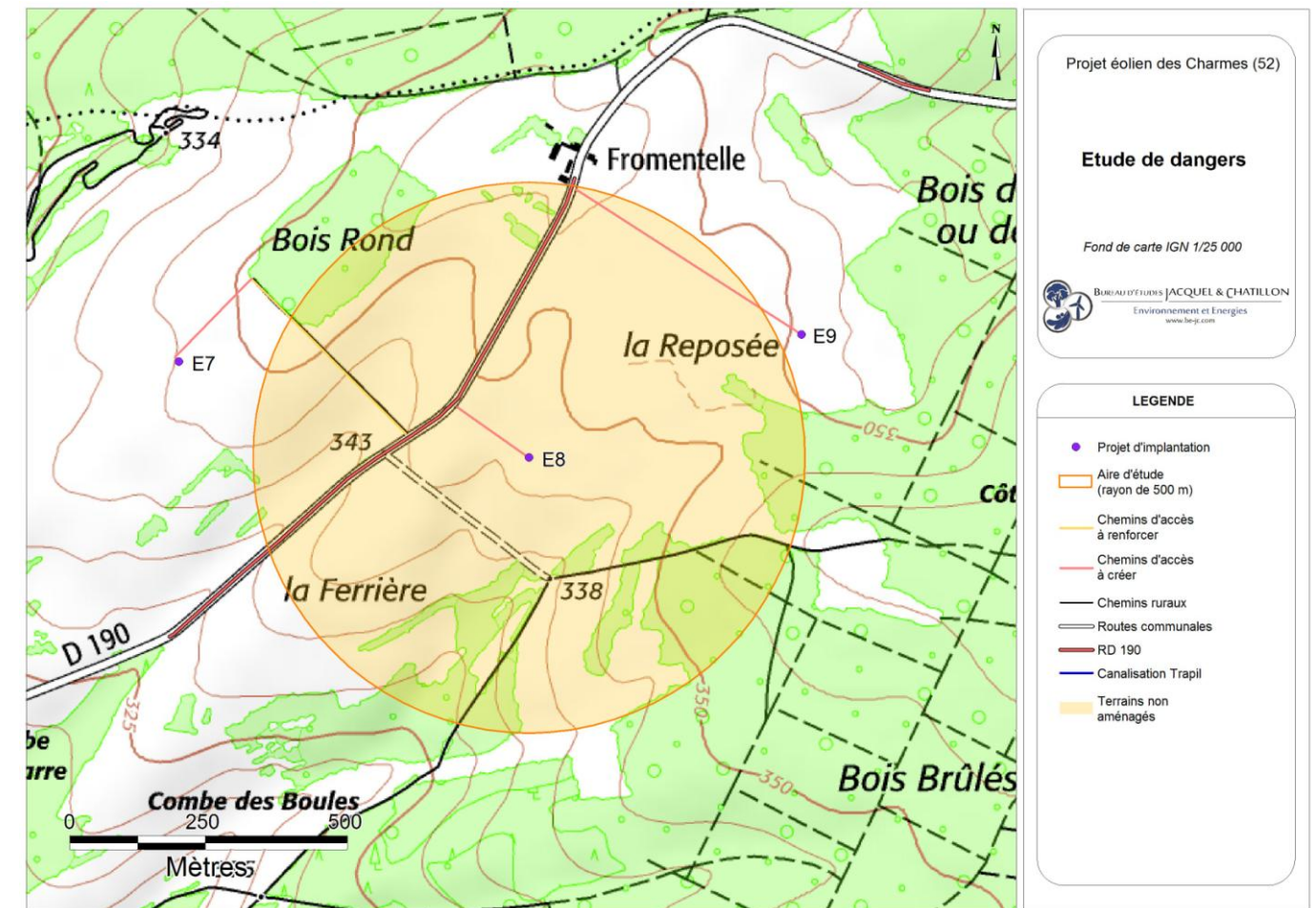
Carte 22 : Éolienne n°8 – Zones à enjeux (Source : BE Jacquel et Chatillon)
