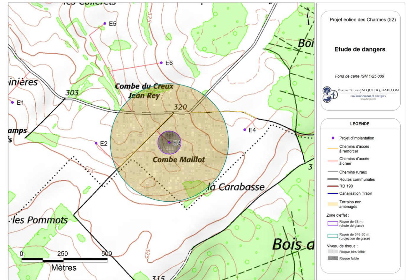
Carte 31 : Éolienne n°3 – Risques liés à la chute et à la projection de glace (Source : BE Jacquiel et Chatillon)
