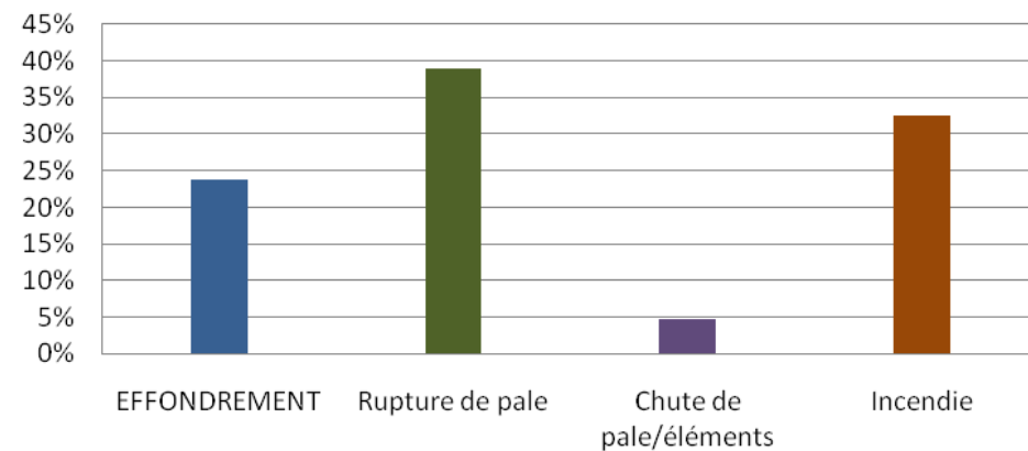
Figure 6 : Répartition des événements accidentels dans le monde entre 2000 et 2011 (Source : INERIS)
