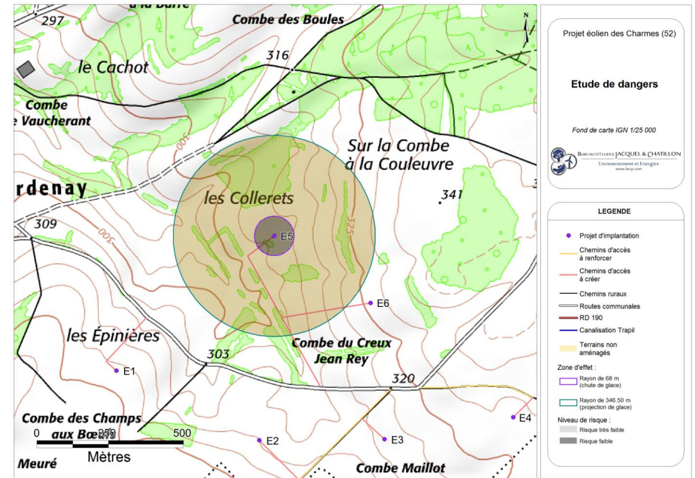
Carte 35 : Éolienne n°5 – Risques liés à la chute et à la projection de glace (Source : BE Jacquiel et Chatillon)
