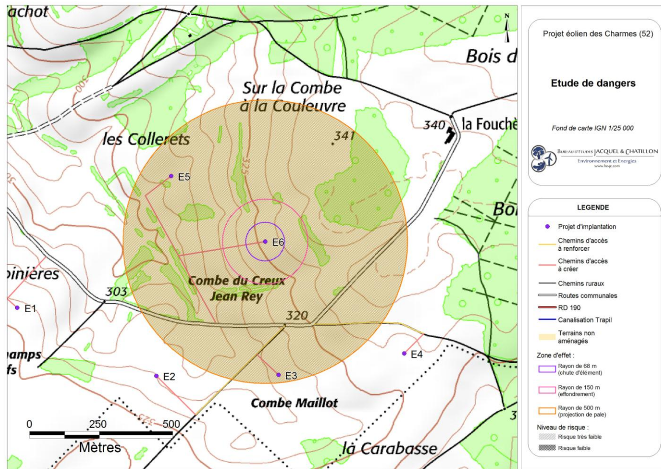
Carte 36 : Éolienne n°6 – Risques liés à l'effondrement de l'éolienne, à la chute d'élément de l'éolienne, et à la projection de pale ou de fragment de pale (Source : BE Jacquel et Chatillon)
