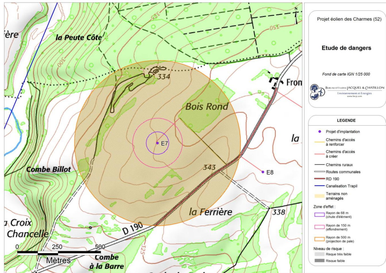
Carte 38 : Éolienne n°7 – Risques liés à l'effondrement de l'éolienne, à la chute d'élément de l'éolienne, et à la projection de pale ou de fragment de pale (Source : BE Jacquiel et Chatillon)
