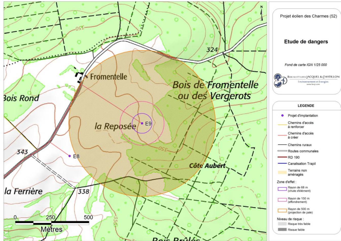
Carte 42 : Éolienne n°9 – Risques liés à l'effondrement de l'éolienne, à la chute d'élément de l'éolienne, et à la projection de pale ou de fragment de pale (Source : BE Jacquiel et Chatillon)
