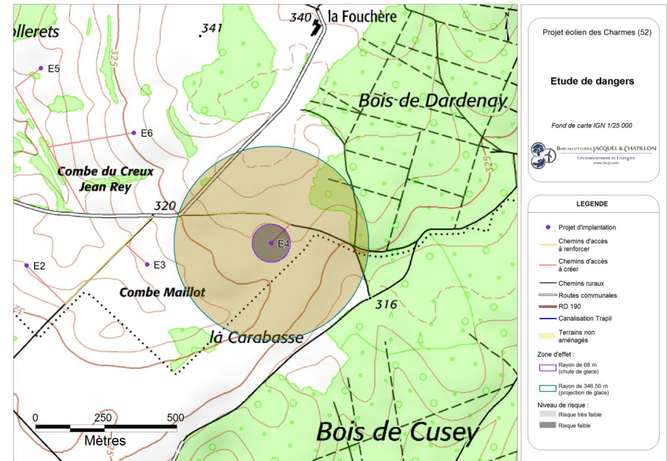
Carte 33 : Éolienne n°4 – Risques liés à la chute et à la projection de glace (Source : BE Jacquel et Chatillon)
