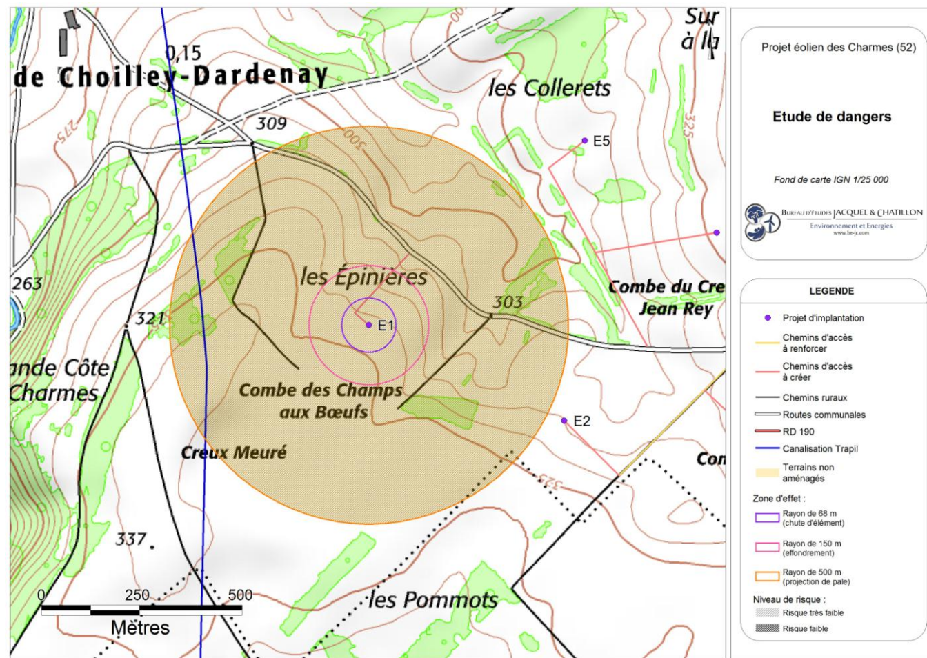
Carte 26 : Éolienne n°1 – Risques liés à l'effondrement de l'éolienne, à la chute d'élément de l'éolienne, et à la projection de pale ou de fragment de pale (Source : BE Jacquel et Chatillon)
