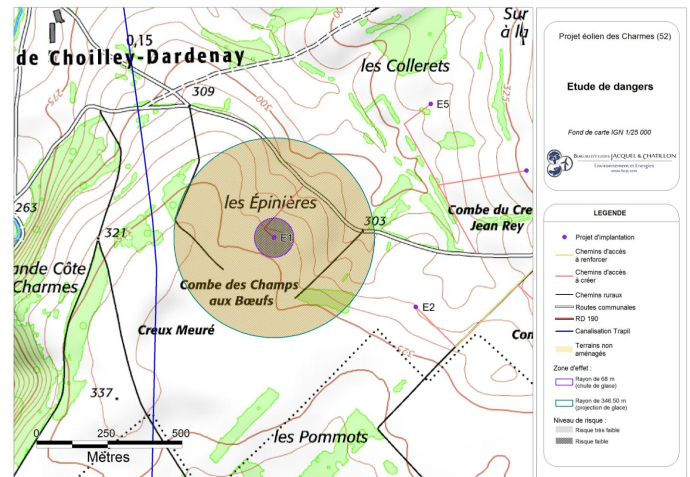
Carte 27 : Éolienne n°1 – Risques liés à la chute et à la projection de glace (Source : BE Jacquel et Chatillon)
