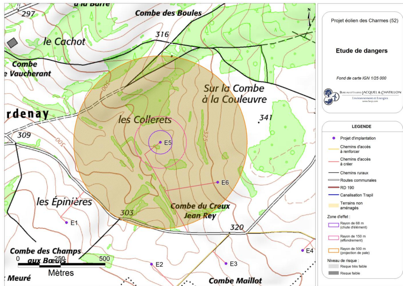
Carte 34 : Éolienne n°5 – Risques liés à l'effondrement de l'éolienne, à la chute d'élément de l'éolienne, et à la projection de pale ou de fragment de pale (Source : BE Jacquiel et Chatillon)
