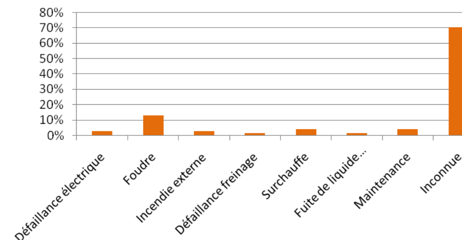
Figure 9 : Répartition des causes premières d'incendie (Source : INERIS)
